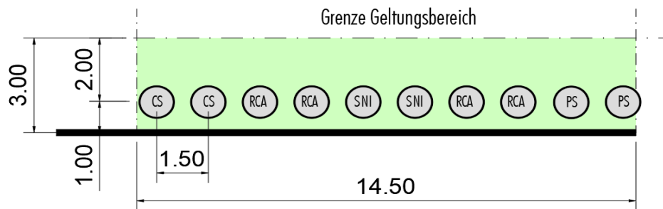
Pflanzschema Eingrünung (Sträucher, 1-reihige Hecke) (14,5 m lang 3,00 mbreit)
