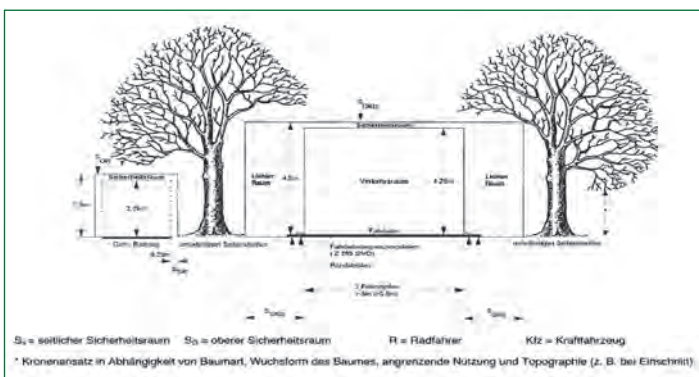
Grafik: Beispielhafte Darstellung des Lichten Raumes in Anlehnung an RAS-Q für anbaufreie Straßen, © Stadt Ellingen (Übermittlung)
