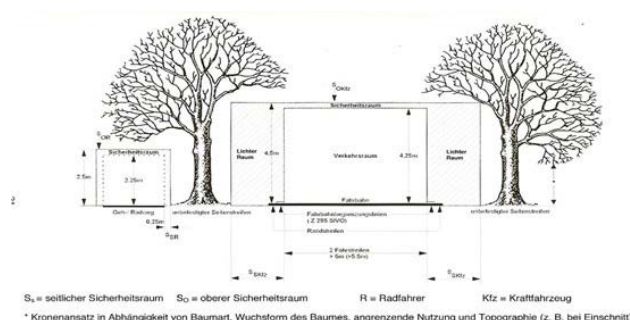
Abb. 2: Beispielhafte Darstellung des Licht Raumes in Anlehnung an RAS-Q für anbaufreie Straßen
